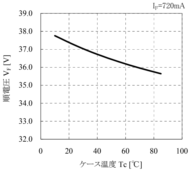
◆ケース温度－順電圧特性
