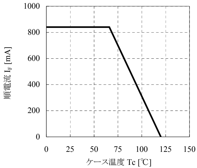
◆ケース温度－順電流定格
