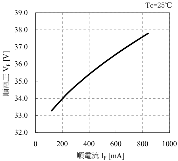
◆順電流－順電圧特性
